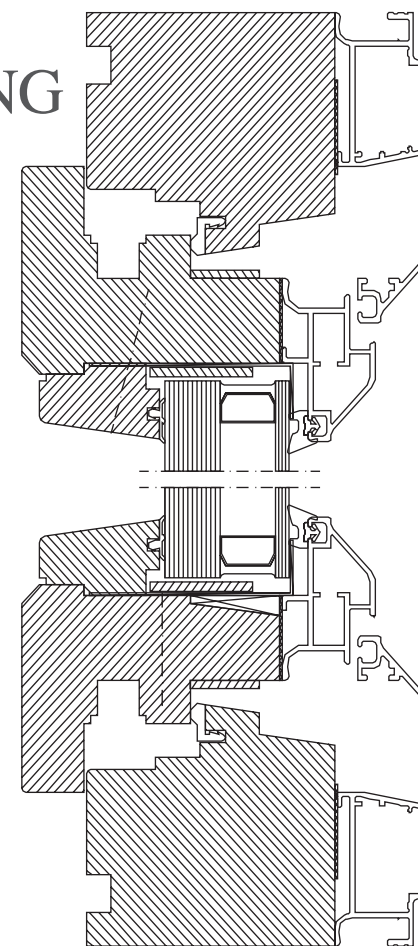
Tegning nr. 7-27-44, vertikalt snitt
