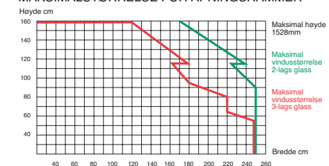
MAKSIMALSTØRRELSE FOR ÅPNINGSRAMMER
